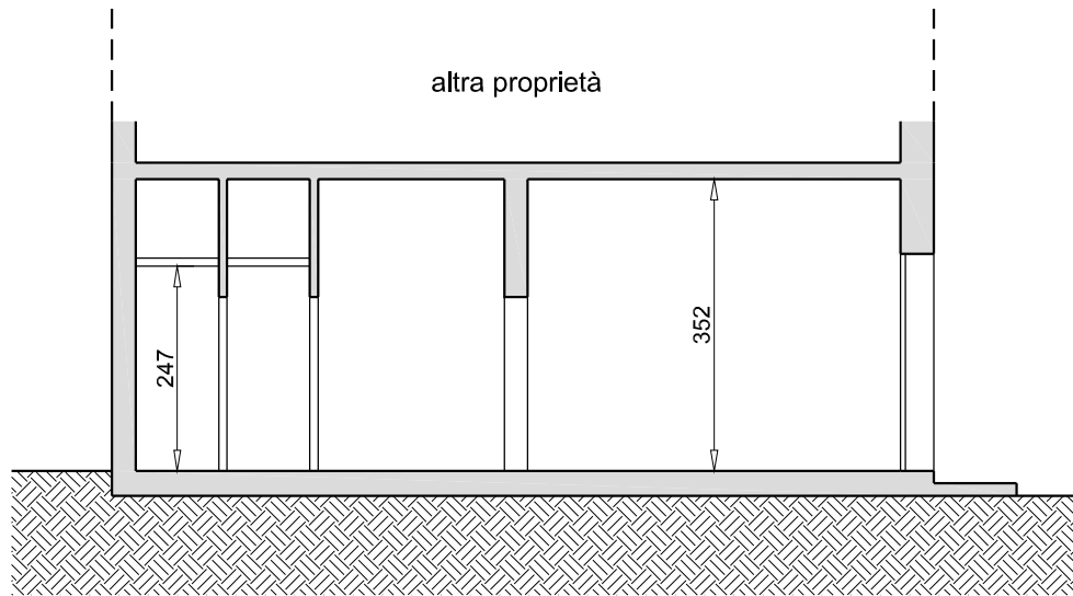
SEZIONE A-A (1:100)
