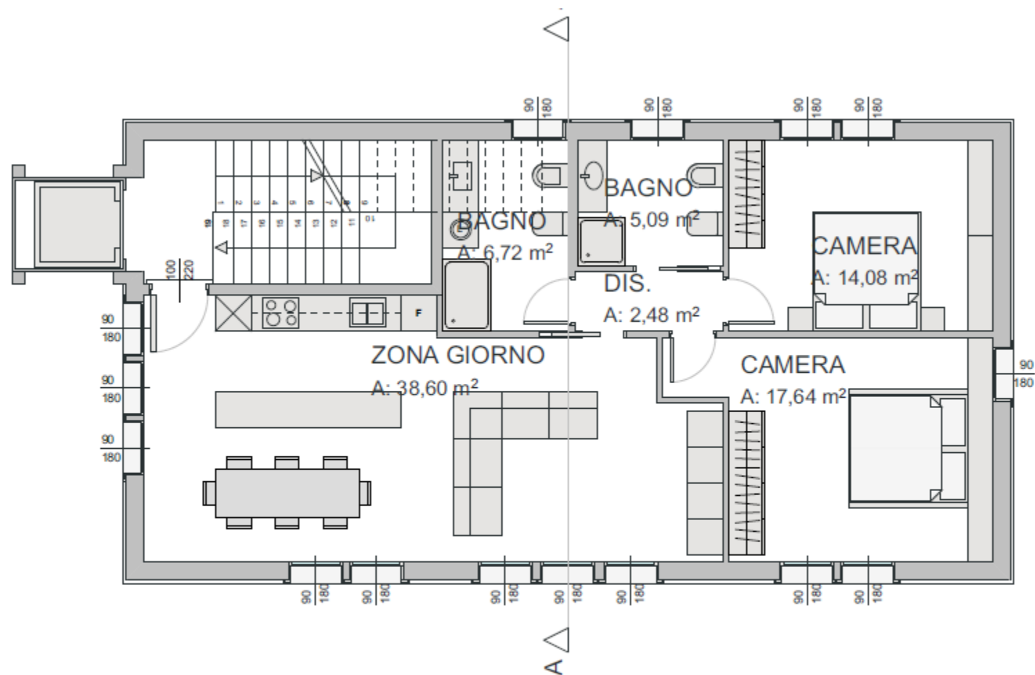
Appartamento p1-2 (versione 2 camere)
